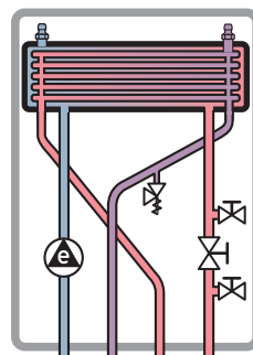
Shematski prikaz
